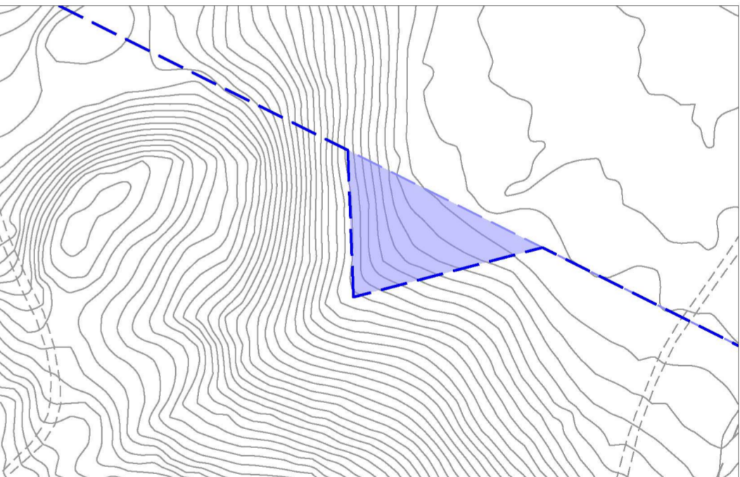
Utvidelse for pistolskytebane (1:1500)
